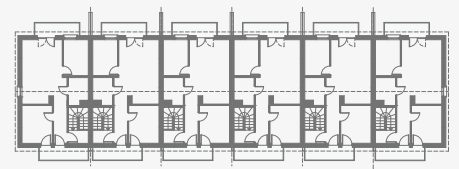
Rzut poddasza
