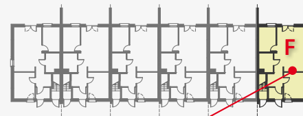
Rzut parteru
